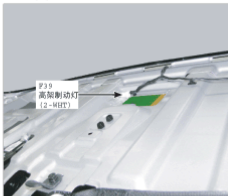
87. 后窗台板
